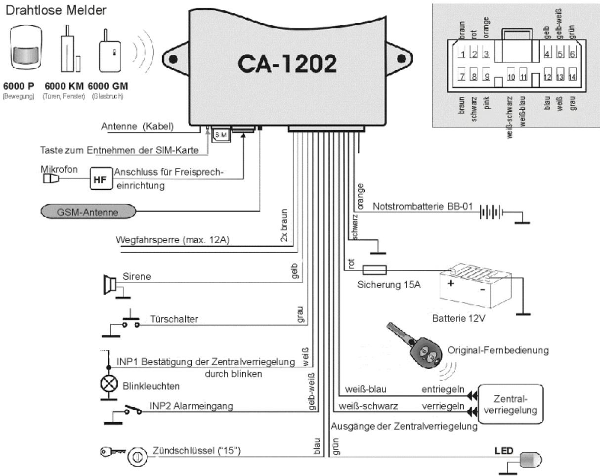
Abb. 1: Installation der Auto alarmanlage in Modus 2
