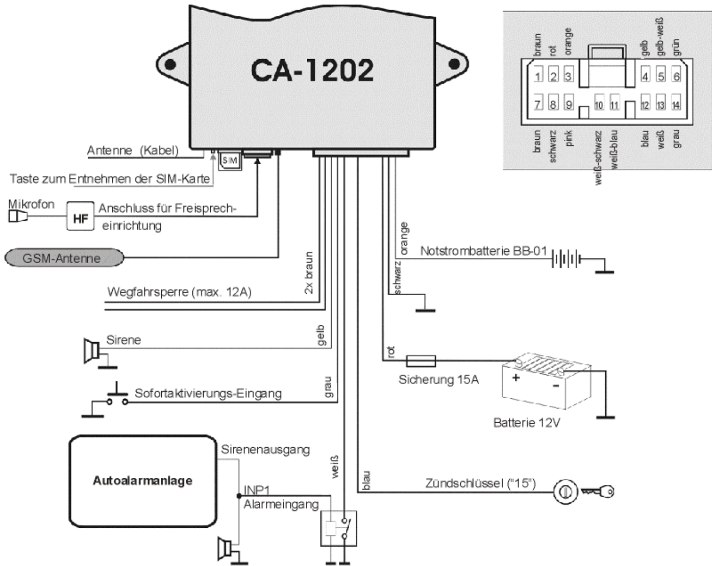
Abb. 1: Installation des GSM-Pagers in Modus 3
